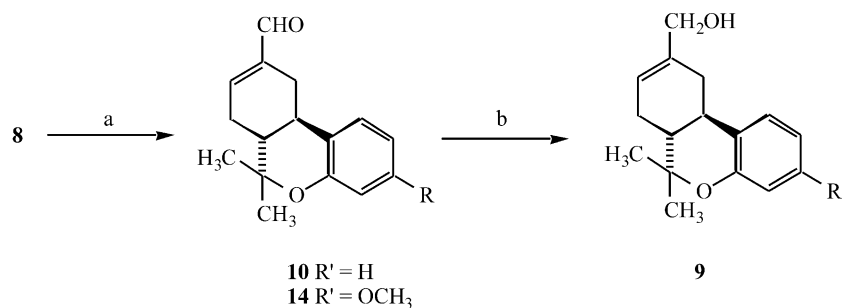
Scheme 1. (a) HOTs/ C_6H_6 , 80 °C; (b) CH_3I/KOH/DMF , 25 °C; (c) NaH/THF , 0 °C then (C_2H_5O)_2P(O)Cl ; (d) Li/NH_3 , THF, -78 °C.
